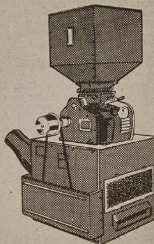
MAQUINARIA Y MOLINOS DE PILAR ARROZ
